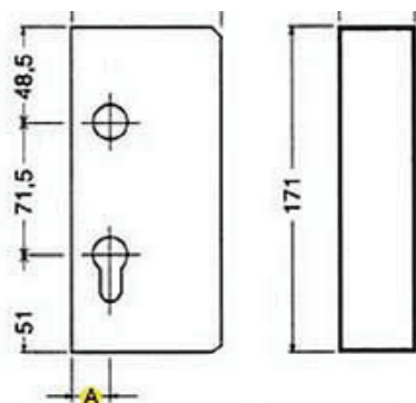
Casetă pentru broască
