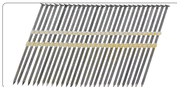
CLOUS BANDE PLASTIQUE 21° STANDARD Intérieur, catégorie de service 1
