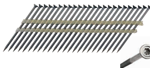
CLOUS BANDE PLASTIQUE 34° ELECTRO-GALV 12µm Extérieur protégé, catégorie de service 2
