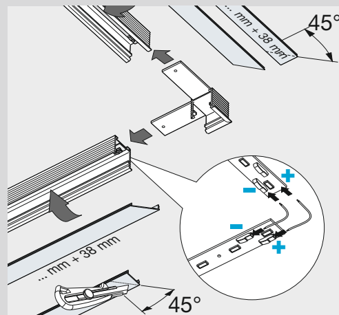
XM2034-U90 Giunzione 90° parete-parete / soffitto-soffitto trim 90° Wall to wall / ceiling to ceiling junction trim
