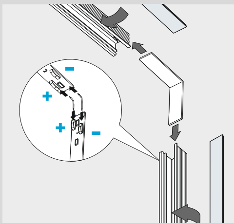
XM2033/34-ANG Giunzione 90° parete-soffitto 90° Wall to ceiling junction
