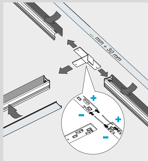
XM2033-UT Giunzione T trimless T junction trimless
