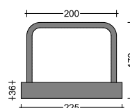
Element dublu-strat Ø 12mm
