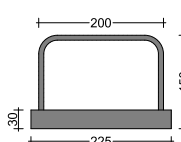
Element dublu-strat Ø 8mm
